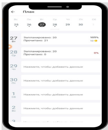
Рисунок 4 – Окно планирования
